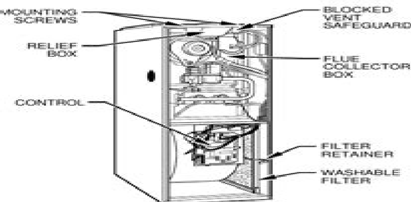
→ Fig. 6—Model 383KAV Upflow
