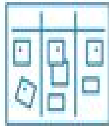
Kanban
