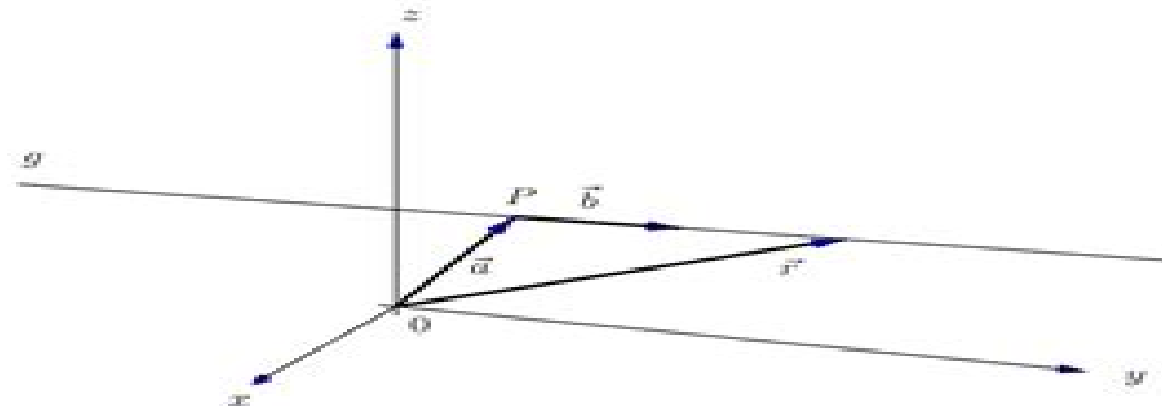
Abb. 2.1: Gerade im \mathbb{R}^3
