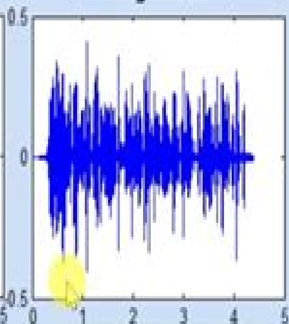
Stego Audio
